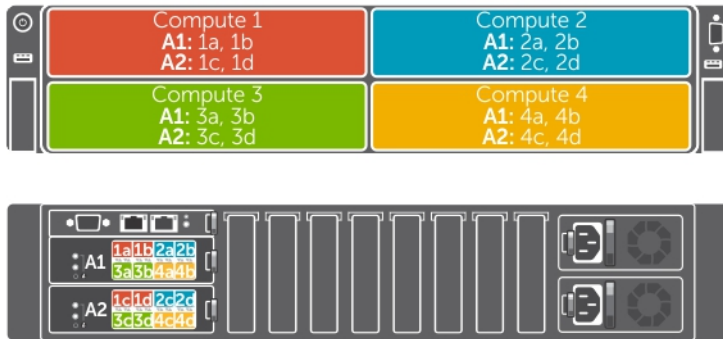
图 9: 增强网络隔离配置的节点到 I/O 模块端口映射
