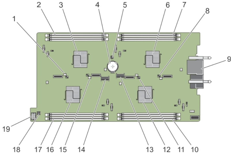
图 31: 系统板连接器
