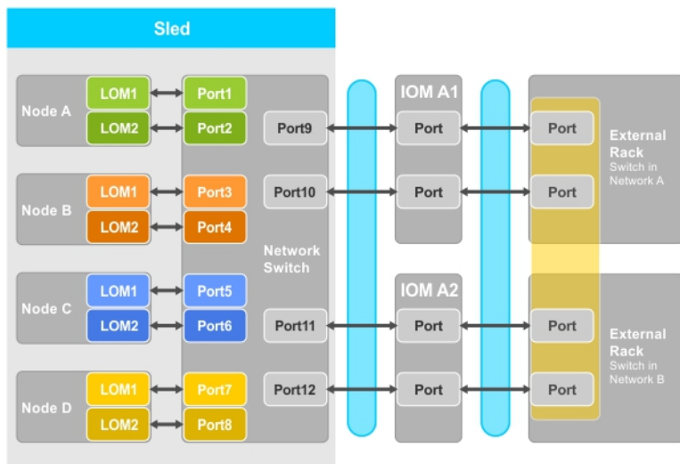
图 6: 网络适配器隔离配置
