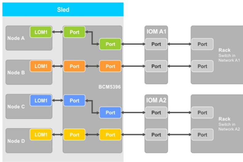
图 8: 增强网络适配器隔离配置
