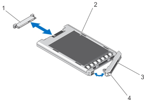
图 22: 卸下和安装 1.8 英寸 SSD
