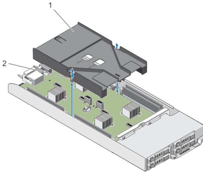
图 14: 卸下和安装冷却导流罩
