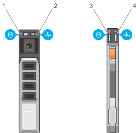
图 3: 硬盘驱动器/SSD 指示灯
