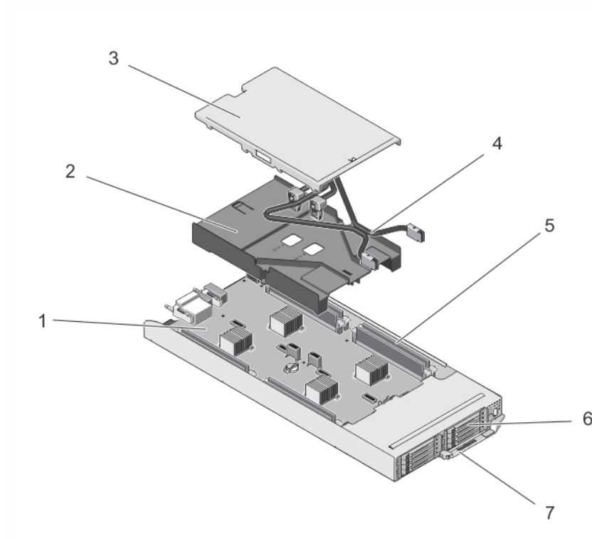
图 12: 底座内部组件 — 1.8 英寸 SSD 系统
