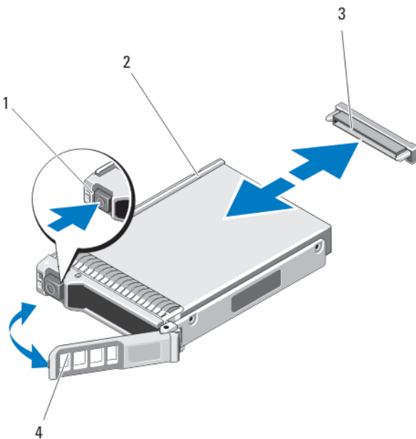
图 21: 卸下和安装 2.5 英寸硬盘驱动器/SSD
