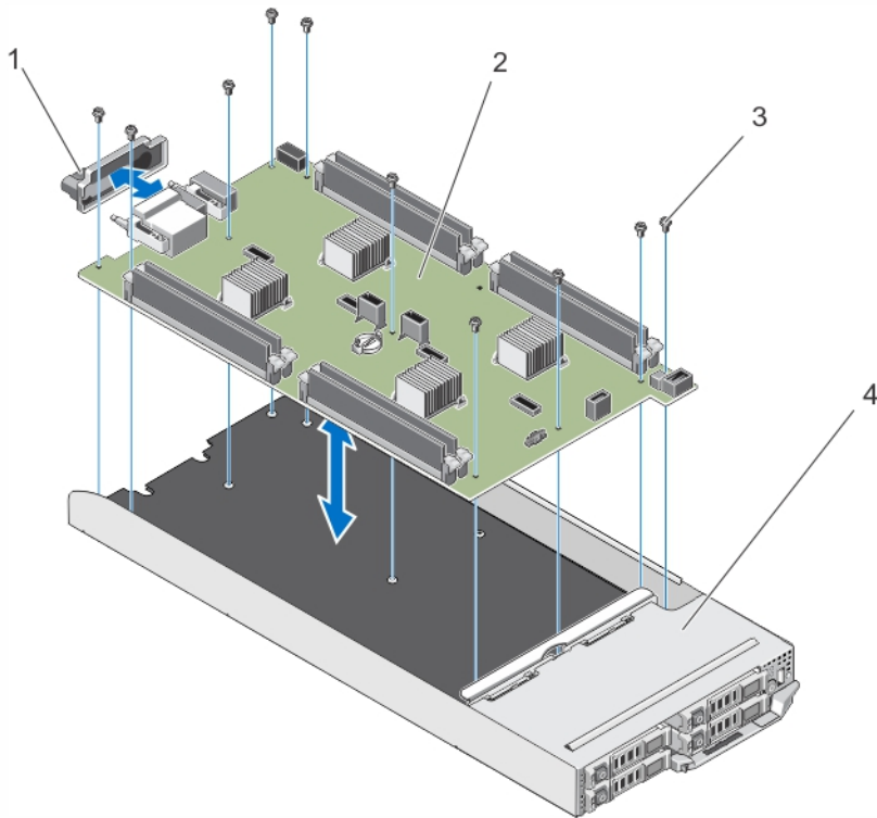
图 29: 卸下和安装系统板
