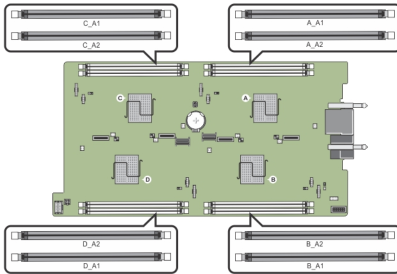
图 15: 内存插槽位置
