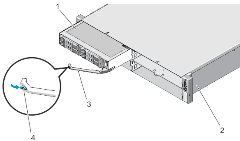
图 10: 卸下和安装底座
