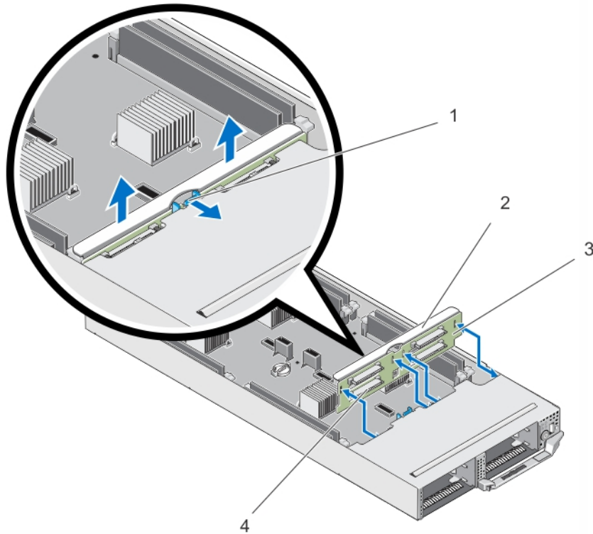
图 25: 卸下和安装硬盘驱动器/SSD 背板
