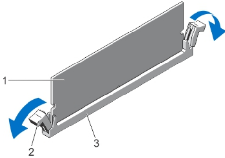
图 16: 弹出内存模块
