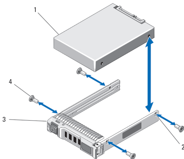
图 23: 在硬盘驱动器/SSD 托盘中卸下和安装 2.5 英寸硬盘驱动器/SSD
