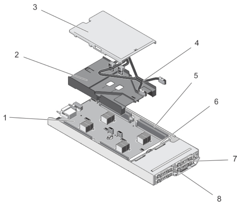
图 11: 底座内部组件 — 2.5 英寸硬盘驱动器/SSD 系统
